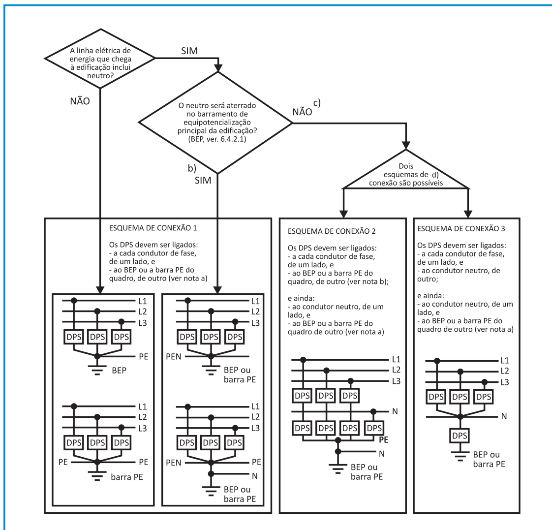
Figura 23 - Esquemas de conexão dos DPS
