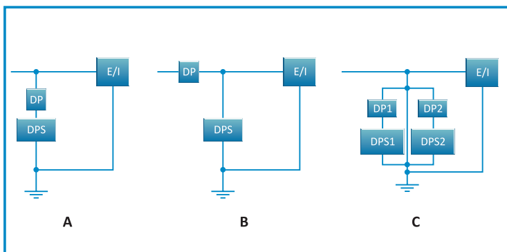
Figura 24 - Esquema de ligação entre DPS, DP e E/I
