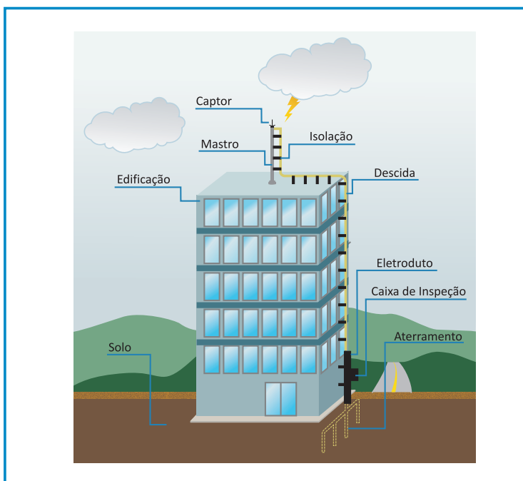
Figura 21 - Exemplo de para-raio do tipo Franklin
