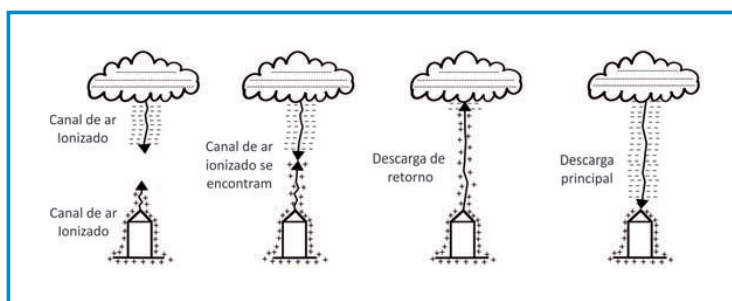
Figura 20 - Esquema de formação do raio
