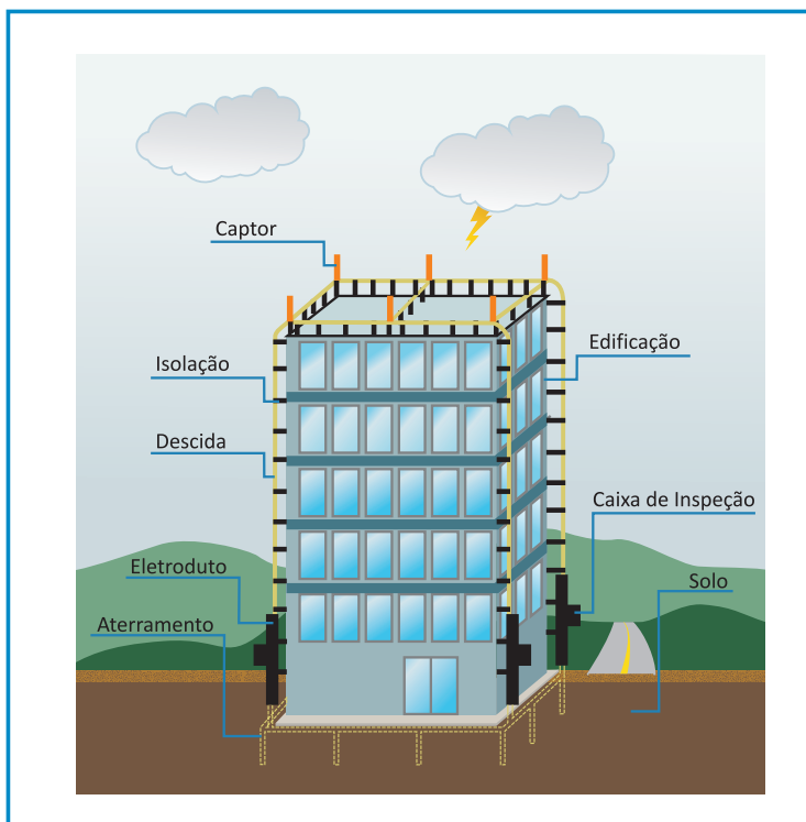
Figura 22 - Exemplo de para-raio do tipo Gaiola de Faraday
