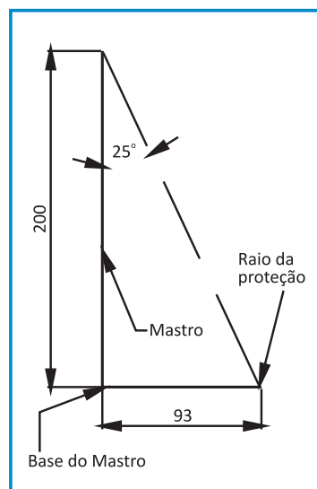
Figura 19 - Exemplo de dimensionamento de captores, método Franklin
