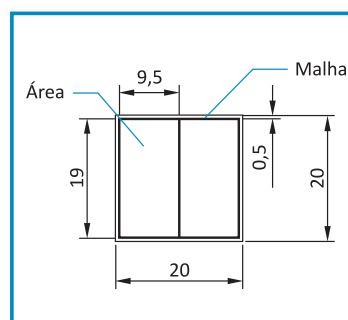
Figura 20 - Exemplo de dimensionamento de captores, método Gaiola de Faraday
