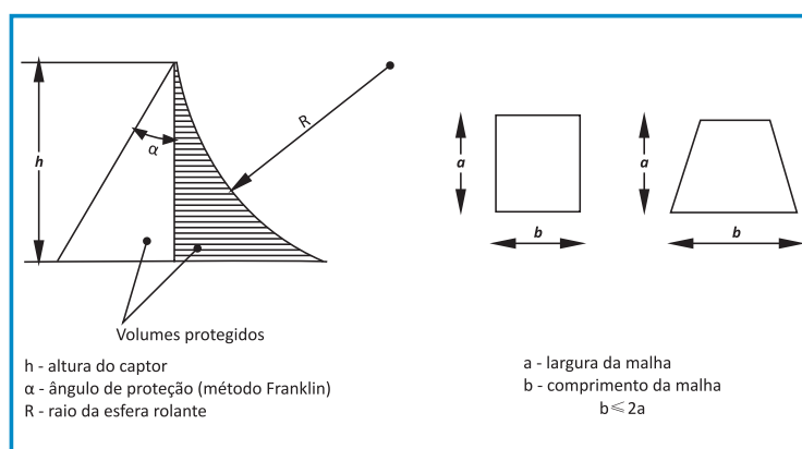
Figura 25 - Parâmetros e volumes de proteção do SPDA
